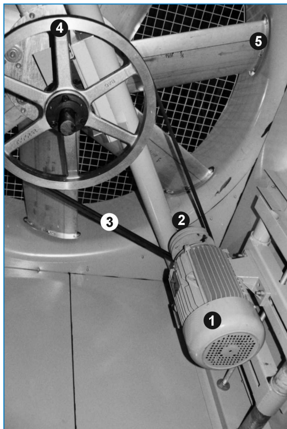
Système d'entraînement
